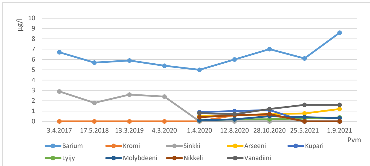
Kuva 8. Vanhemman tuhkatien laskuojan vesinäytteistä määritetyt metallipitoisuudet.
