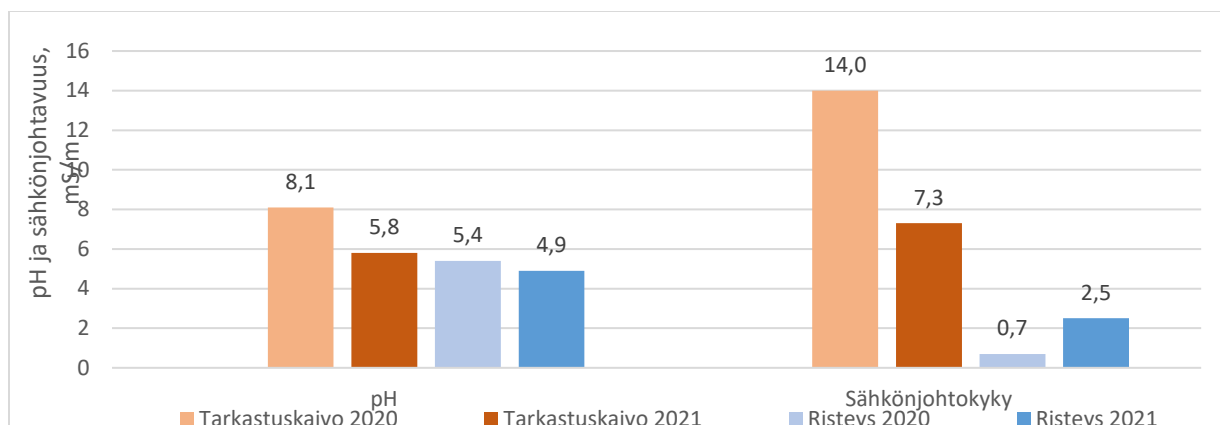
Kuva 9. Vanhemman tiekohteen maanäytteiden pH ja sähkönjohtokyky.
