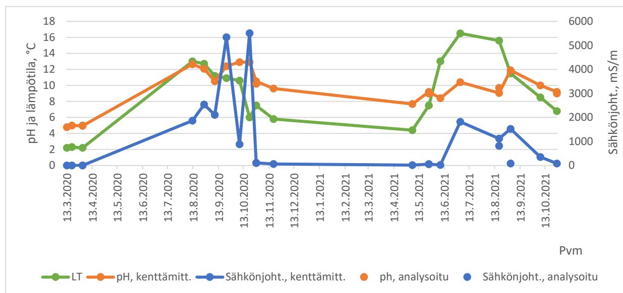
Kuva 12. Uudemman tiekohteen ojaveden laboratorioanalyysien ja kenttämittausten tulokset.
