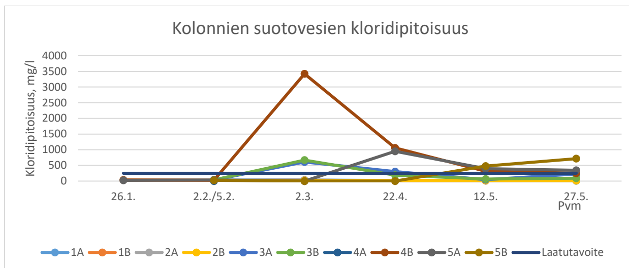
Kuva 24. Kolonnien suotovedestä mitatut kloridipitoisuudet.
