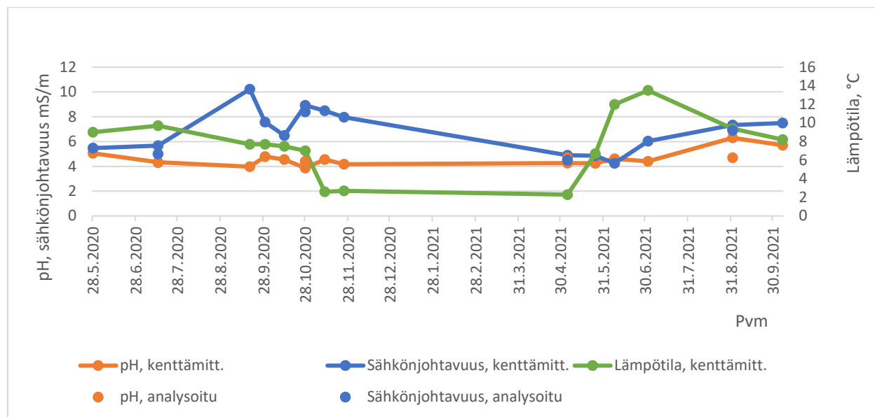
Kuva 18. Tuhkalannoituskohteen ojaveden laboratorioanalyysien ja kenttämittausten tulokset.
