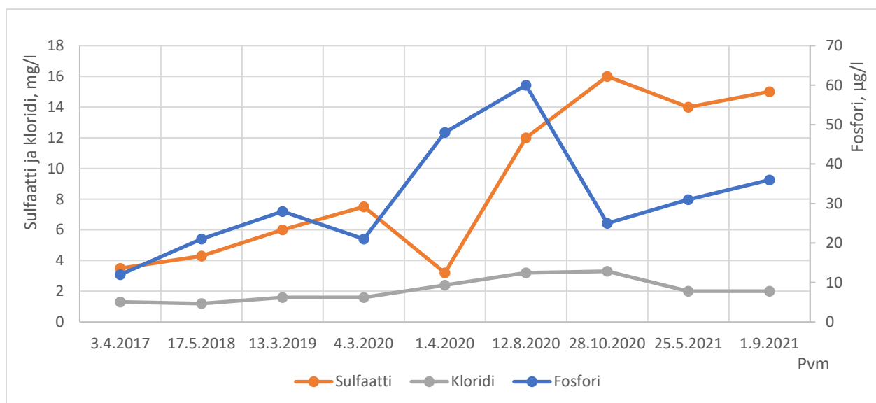
Kuva 7. Tuhkatien laskuojan vesinäytteistä määritetyt fosforin (µg/l), sulfaatin (mg/l) ja kloridin (mg/l) pitoisuudet.
