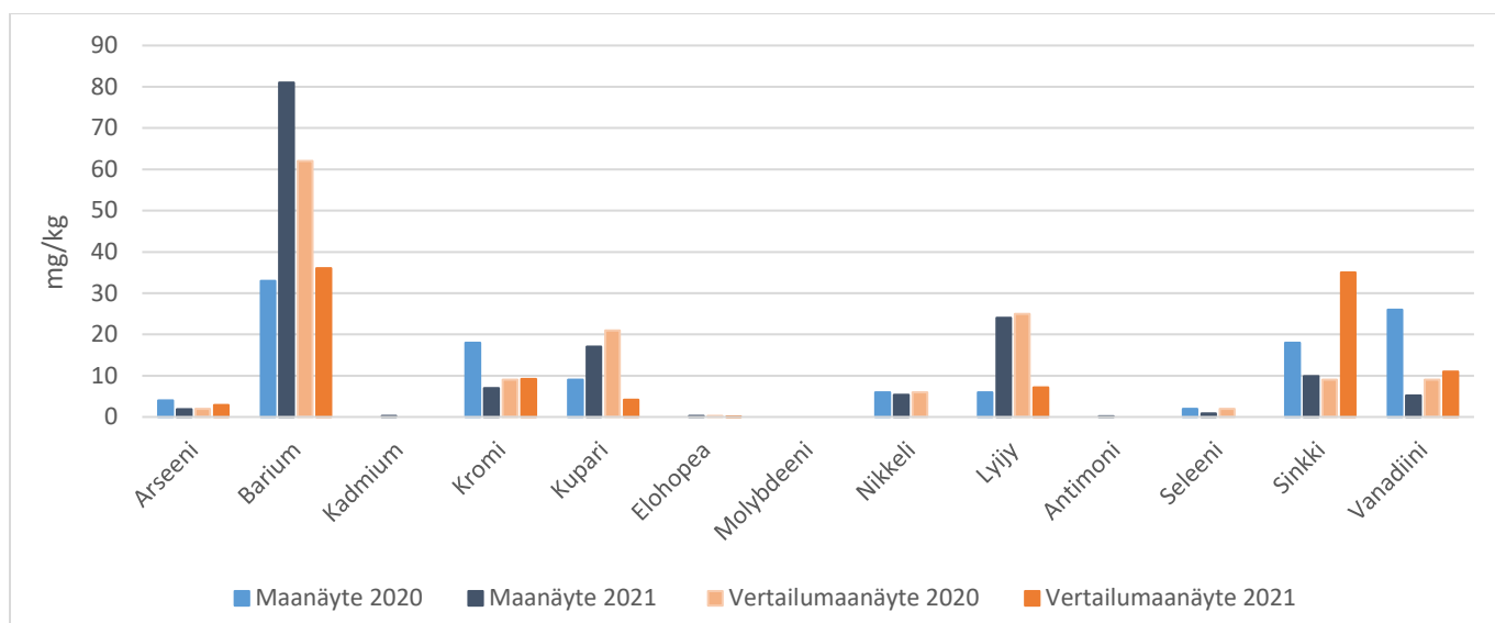
Kuva 17. Uudemman tiekohteen maanäytteiden raskasmetallipitoisuuksien muutos vuodesta 2020 vuoteen 2021.
