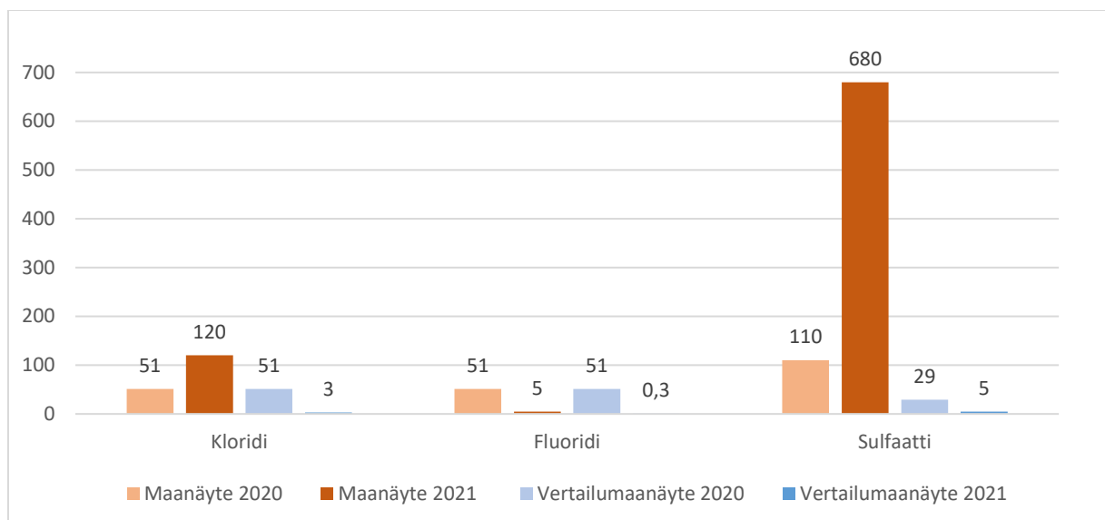
Kuva 16. Uudemman tiekohteen maanäytteiden kloridi-, fluoridi- ja sulfaattipitoisuuksien muutos vuodesta 2020 vuoteen 2021.
