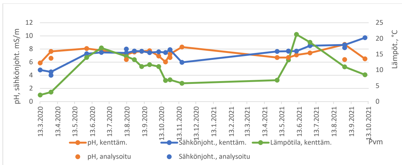
Kuva 6. Vanhemman tiekohteen ojaveden laboratorioanalyysien ja kenttämittausten tulokset.
