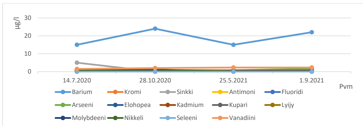
Kuva 20. Tuhkalannoituskohteen metsäojan vesinäytteistä määritetyt raskasmetallipitoisuudet.
