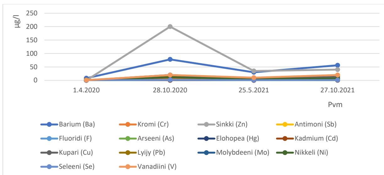
Kuva 14. Uudemman tuhkatie laskuojan vesinäytteistä määritetyt metallipitoisuudet.
