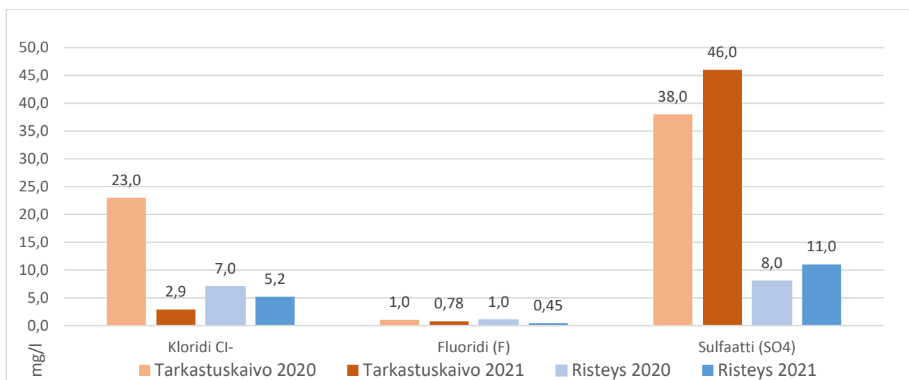
Kuva 10. Vanhemman tiekohteen maanäytteiden kloridi-, fluoridi- ja sulfaattipitoisuudet.
