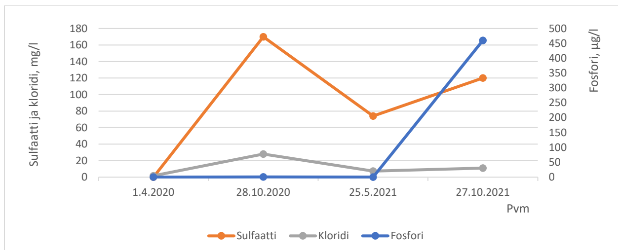
Kuva 13. Tuhkatien laskuojan vesinäytteistä määritetyt fosforin (µg/l), sulfaatin (mg/l) ja kloridin (mg/l) pitoisuudet.
