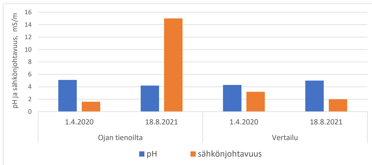
Kuva 15. Uudemman tiekohteen maanäytteistä määritetyt pH- ja sähkönjohtavuusarvot.
