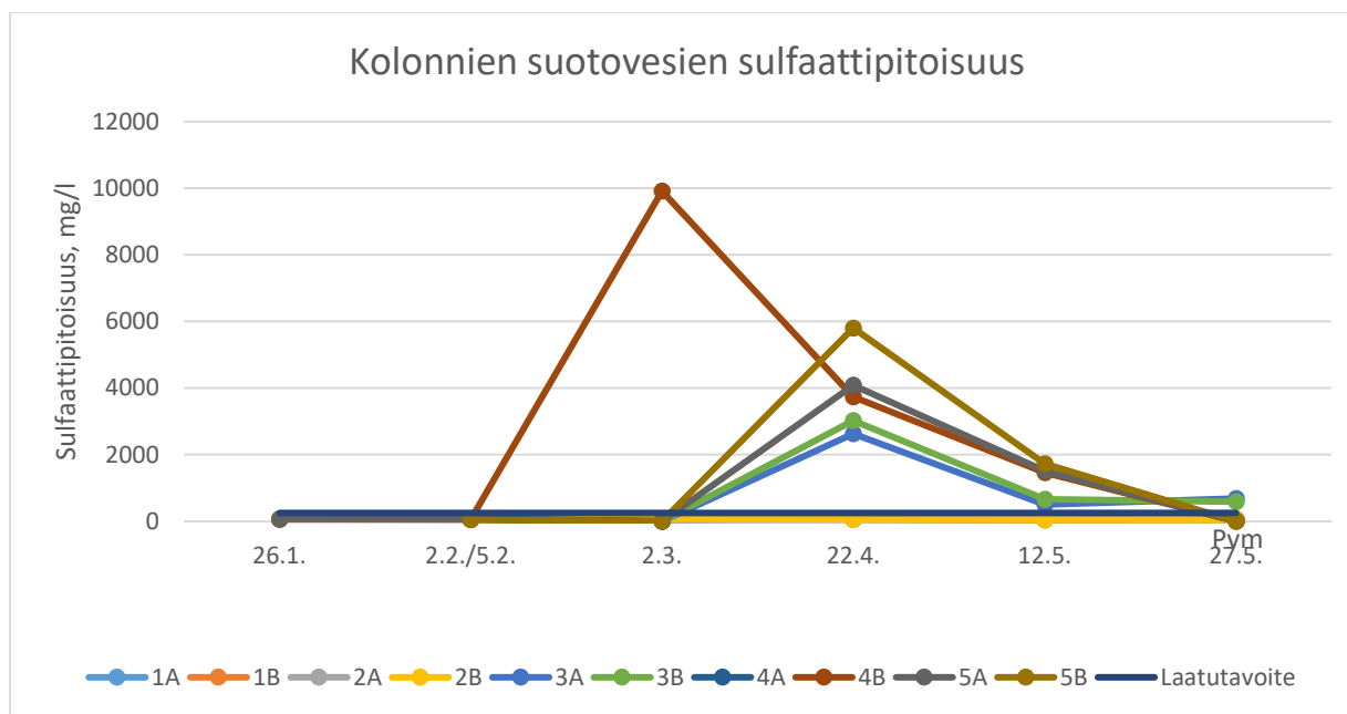
Kuva 23. Kolonnien suotovedestä mitatut sulfaattipitoisuudet.
