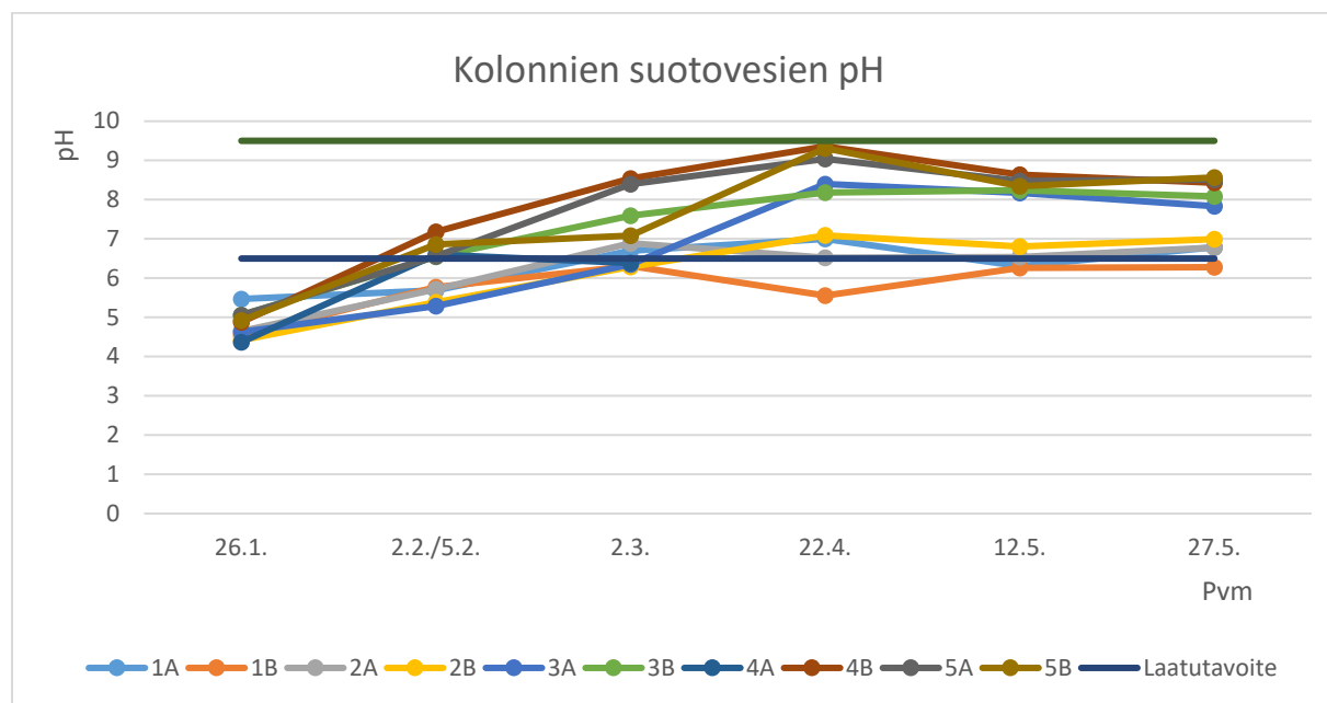
Kuva 21. Tiekolonnikokeen suotovesien pH:n mittaustulokset.
