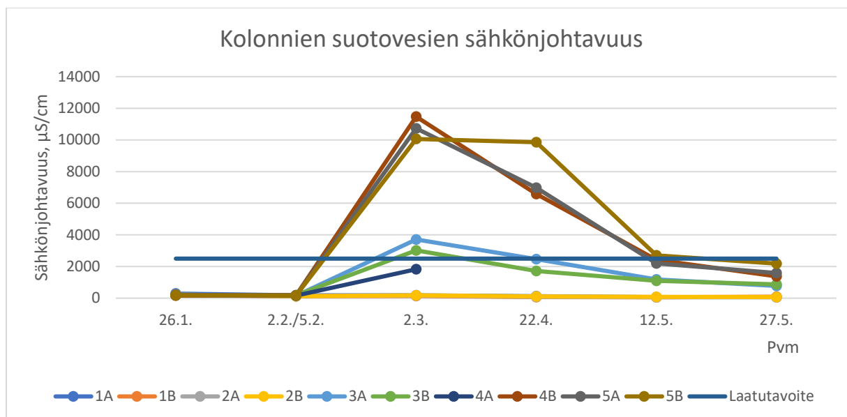
Kuva 22. Kolonnien suotovedestä mitattu sähkönjohtavuus.
