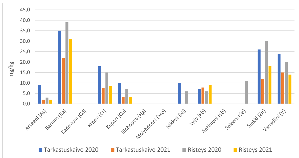
Kuva 11. Vanhemman tiekohteen maanäytteiden metallipitoisuudet.
