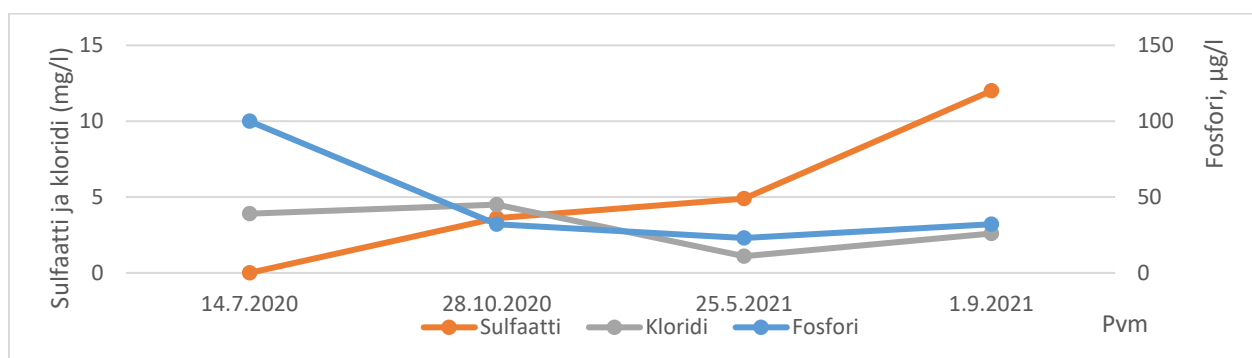
Kuva 19. Tuhkalannoituskohteen ojan vesinäytteistä määritetyt fosforin (µg/l), sulfaatin (mg/l) ja kloridin (mg/l) pitoisuudet.
