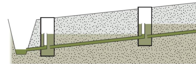
Säätösalaajituksen periaatekuva.
